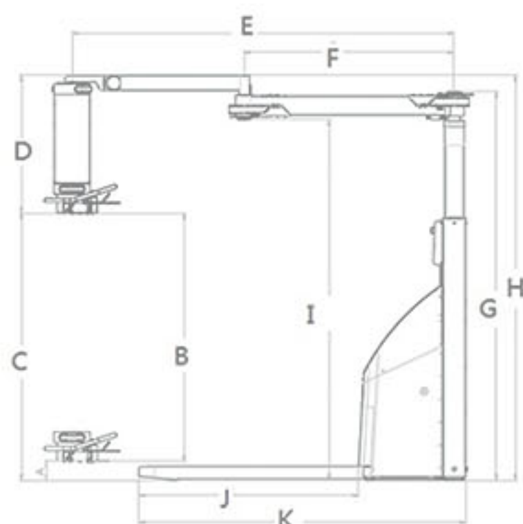
側面圖
